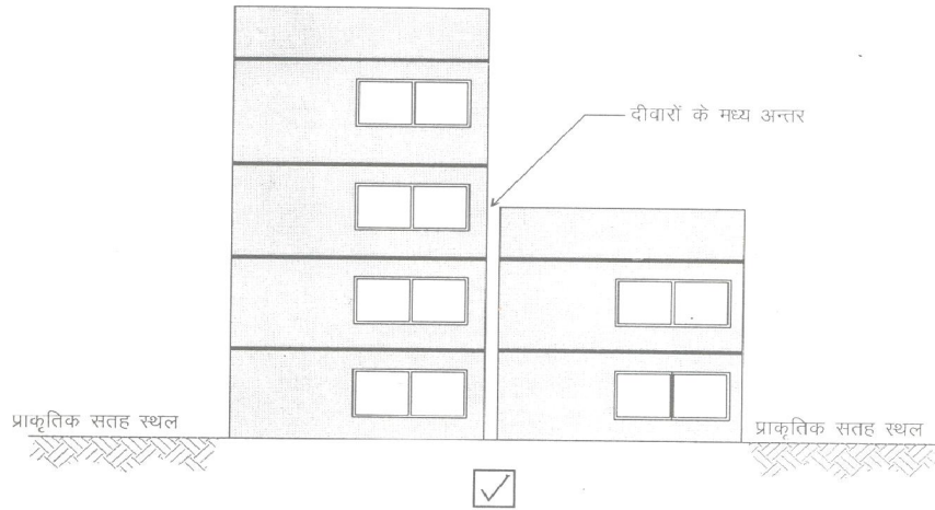
एक दूसरे से लगी हुई संरचनाओं में अलगाव होना चाहिए चित्र क्रमांक 5.6
