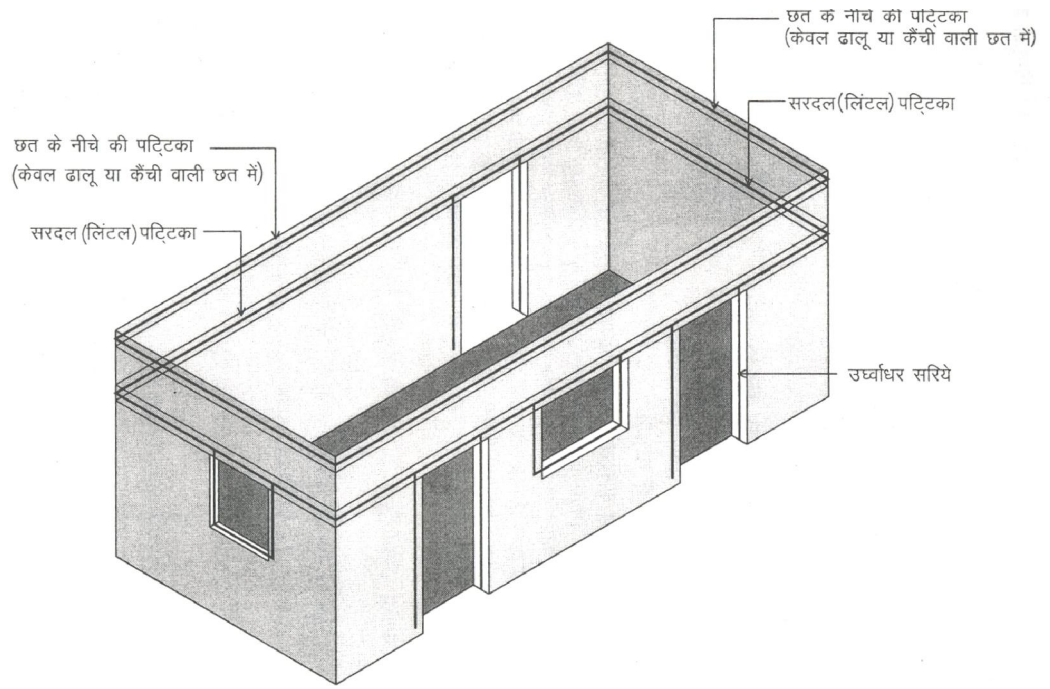
ईट की चिनाई के मकान में भूकंपीय प्रबलन हेतु सरियों के विवरण का विस्तृत चित्रण
